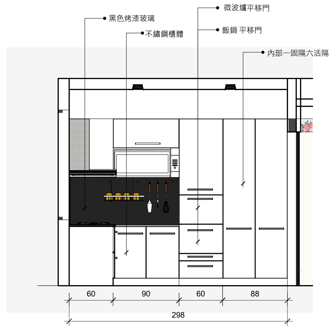
G2立面圖
