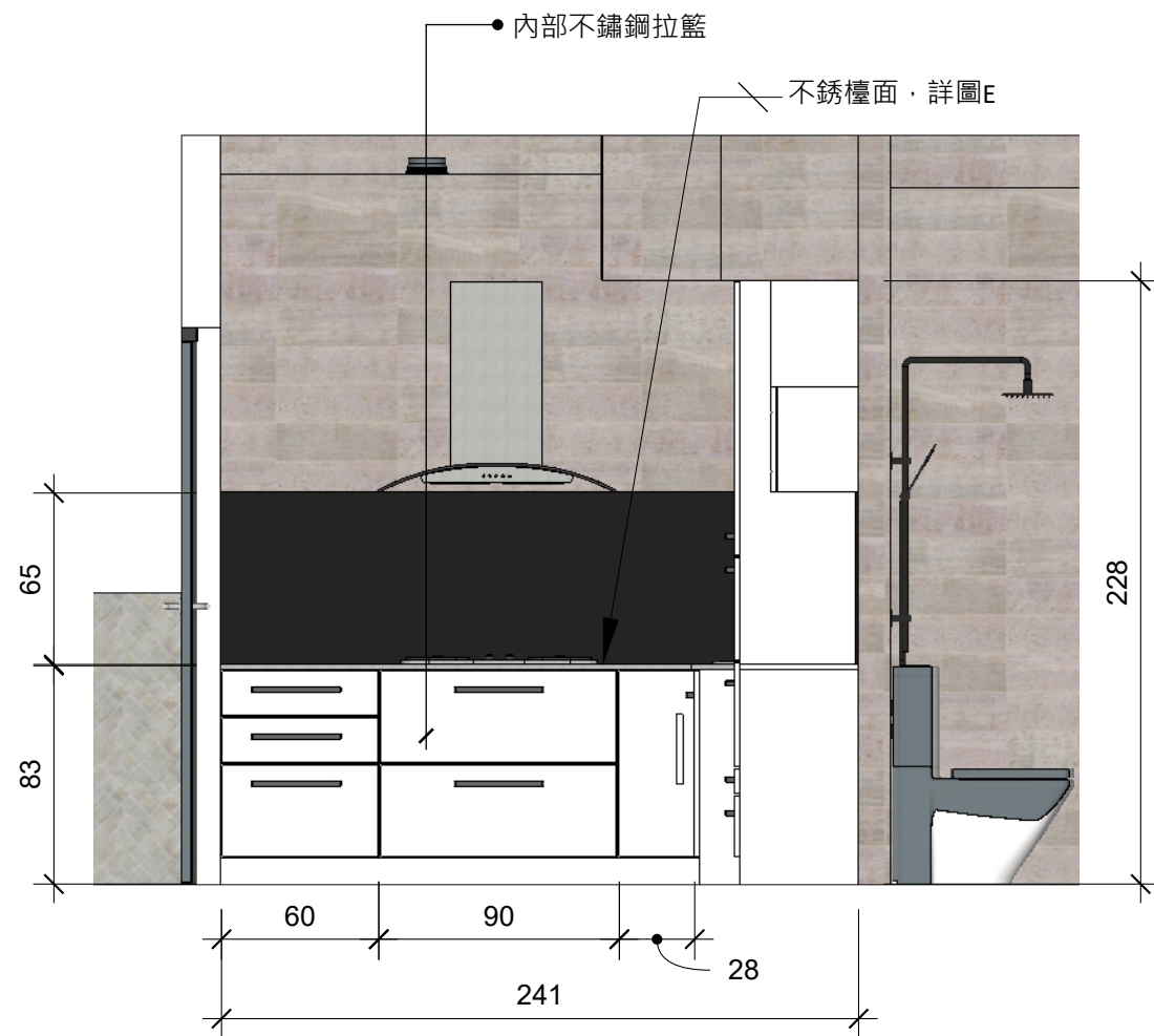
G1立面圖
