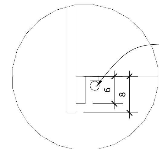
詳圖B: 門片前緣施工大樣圖 比例: 1/5
