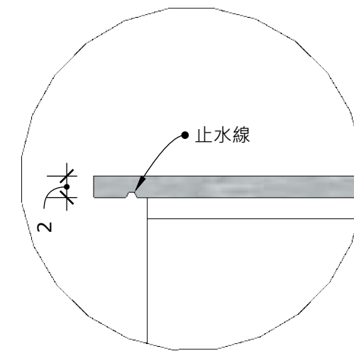
詳圖E: 不鏽鋼檯面施工大樣 比例: 1/5
