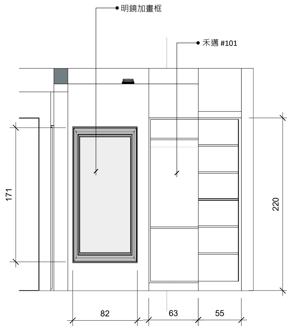
C6立面圖
