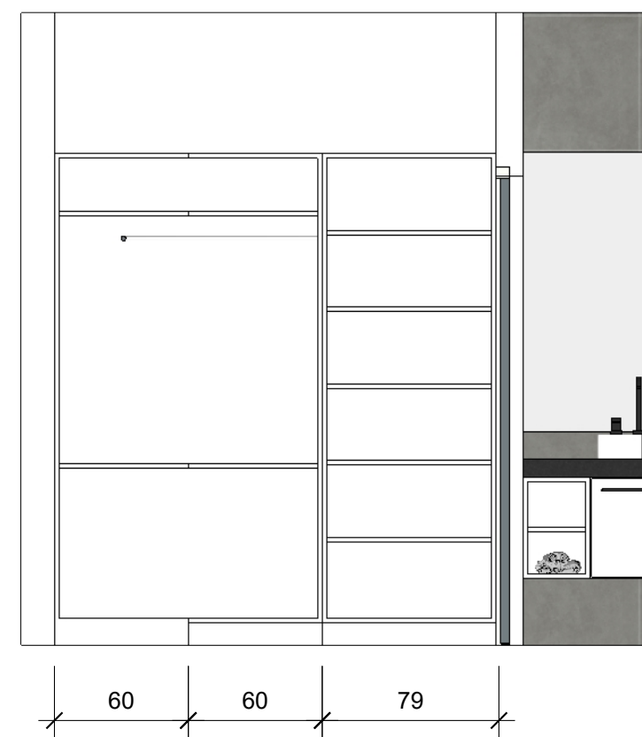
C5立面圖
