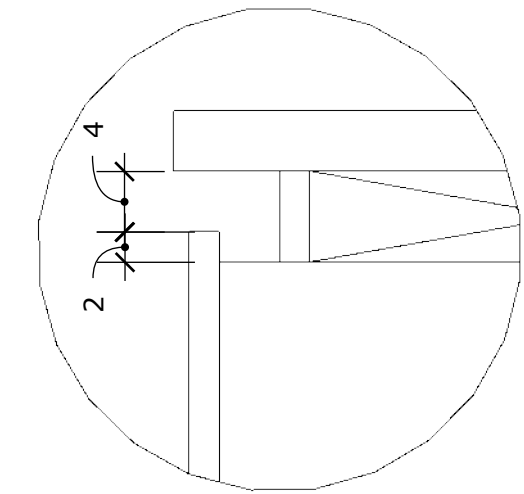
詳圖A: 抽屜前緣施工大樣 比例: 1/5
