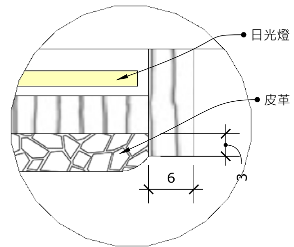
詳圖D: 床頭施工大樣 比例: 1/5
